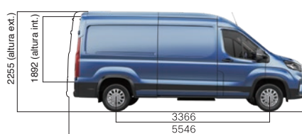
DISTANCIA ENTRE EJES MEDIA, TECHO MEDIO
