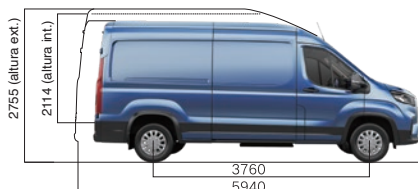
DISTANCIA ENTRE EJES LARGA, TECHO ALTO
